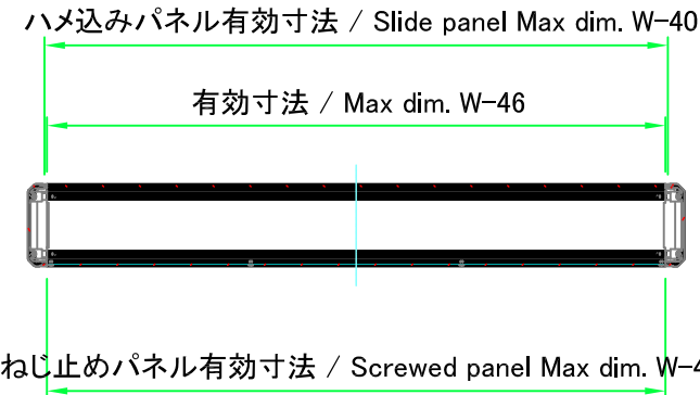
A-A ( 1 : 10 )
