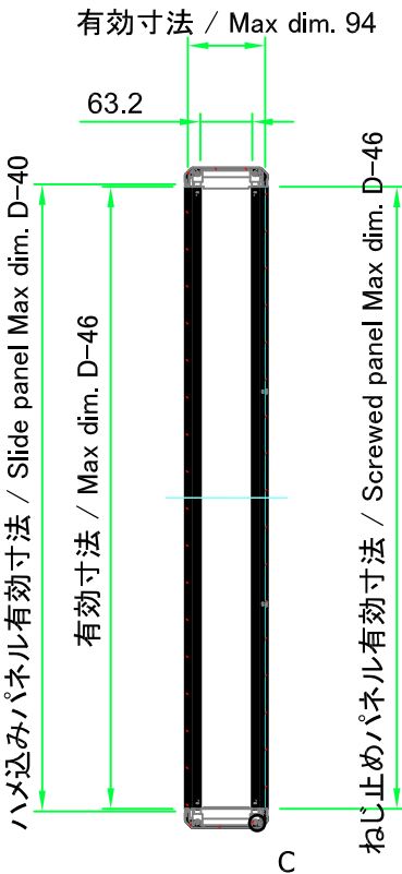
B-B ( 1 : 10 )
